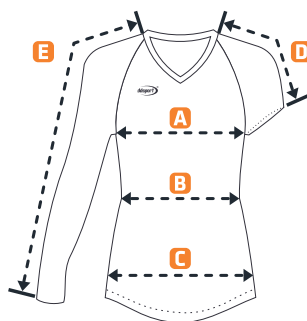
Střih raglán
